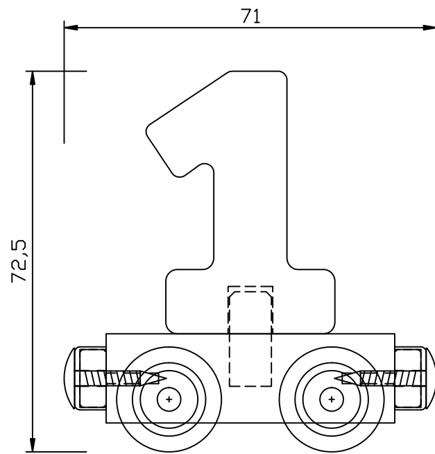
车厢1
