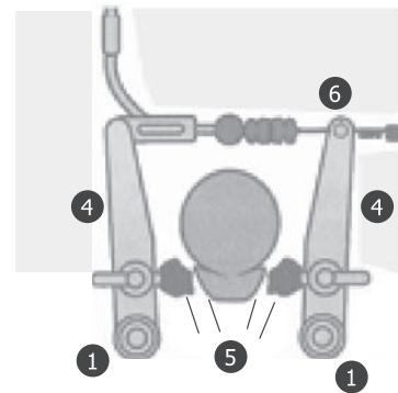
V Brake
